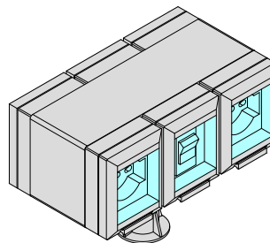
MA90805i 4 Prese Schuko 220V-16A e 2 interruttori magnetotermici 4 Schuko 220V-16A sockets 2 magnetothermic switches
