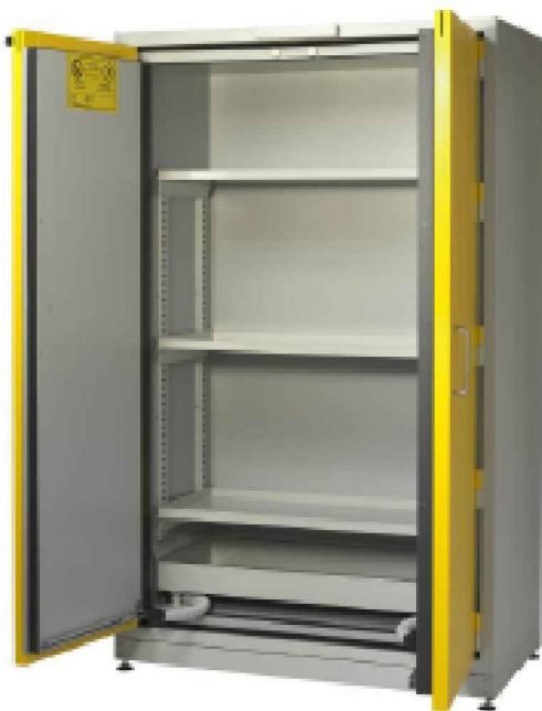
AC 1200CM Armadio per infiammabili - 160 litri Safety storage cabinet - 160 liters L 118 - P 65 - H 198,5 Peso / Weight : 490 KG
