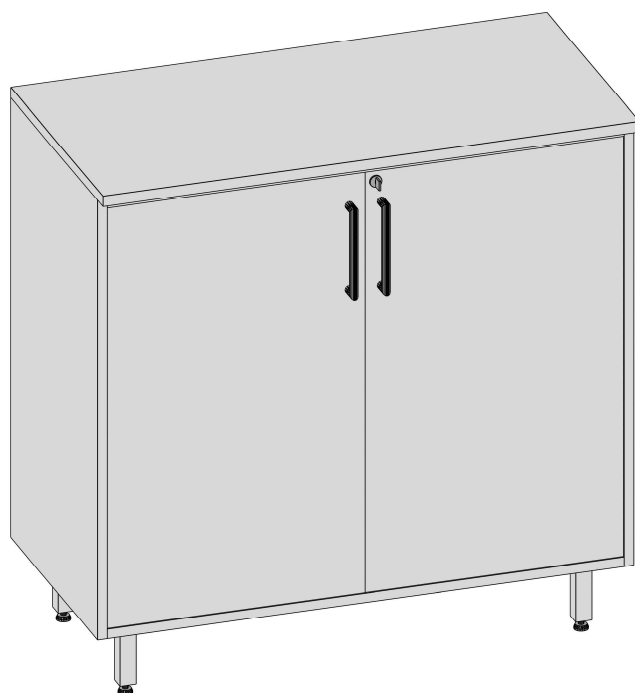
MA903175 - l 100 x p 50 x h 101 Ante battenti cieche / Swing doors
