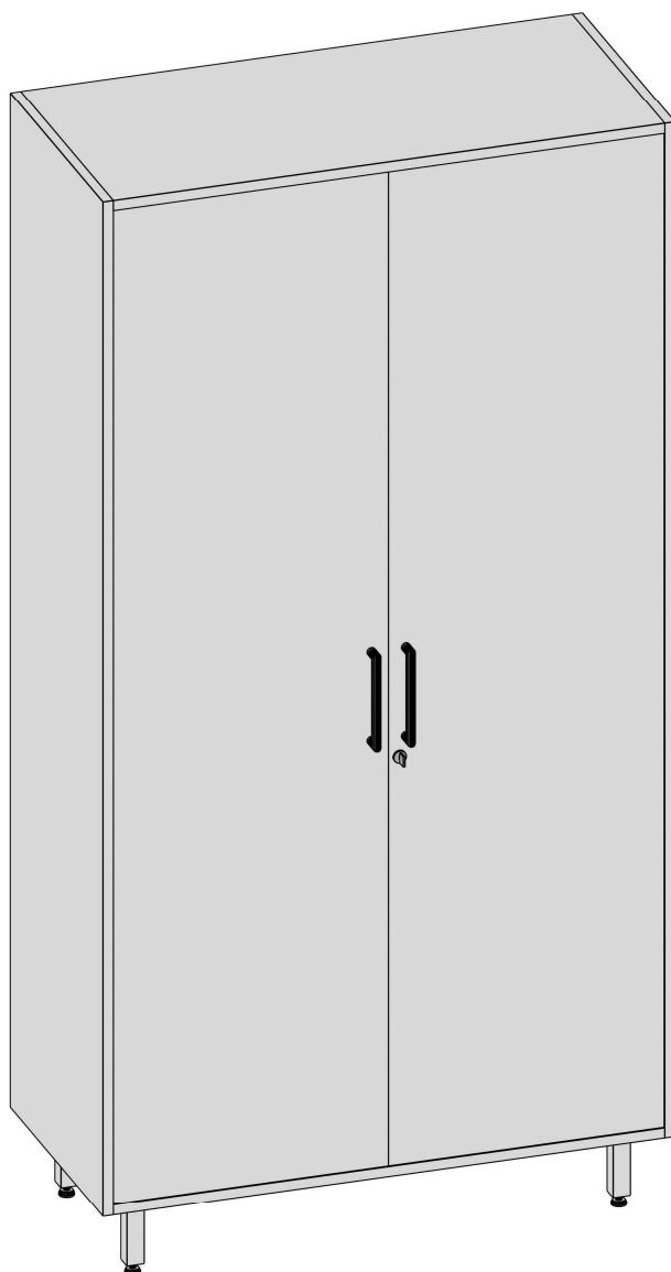
MA903700 - l 100 x p 47 x h 200 Ante battenti cieche / Swing doors
